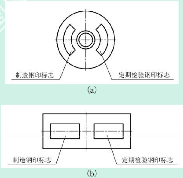
图 D-1 钢印标志位置示意图
